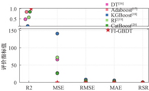
图 2 模型评价指标对比
