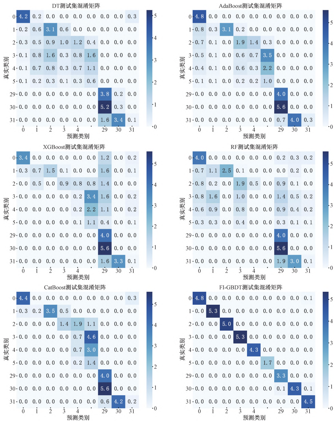
图4 测试集混淆矩阵结果对比
