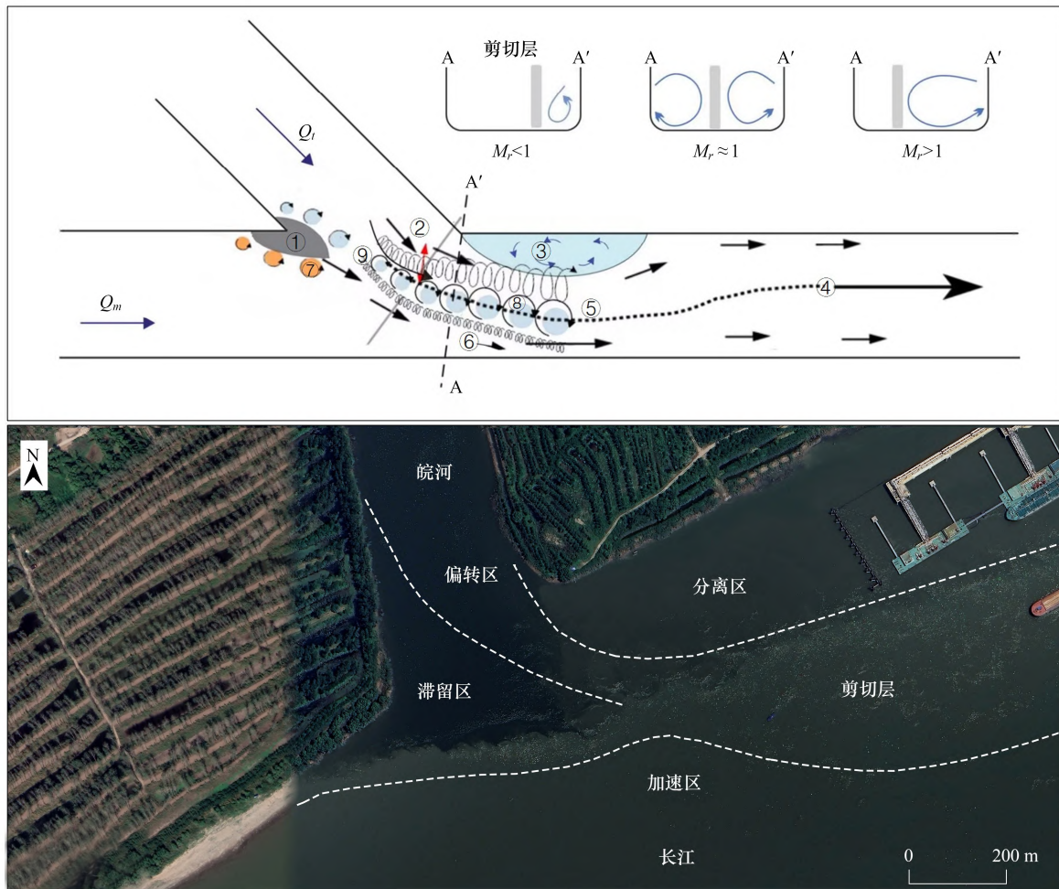
图2 汇流水力区流态、二次流示意图及皖河口流态实际表征 [25,52-53]
